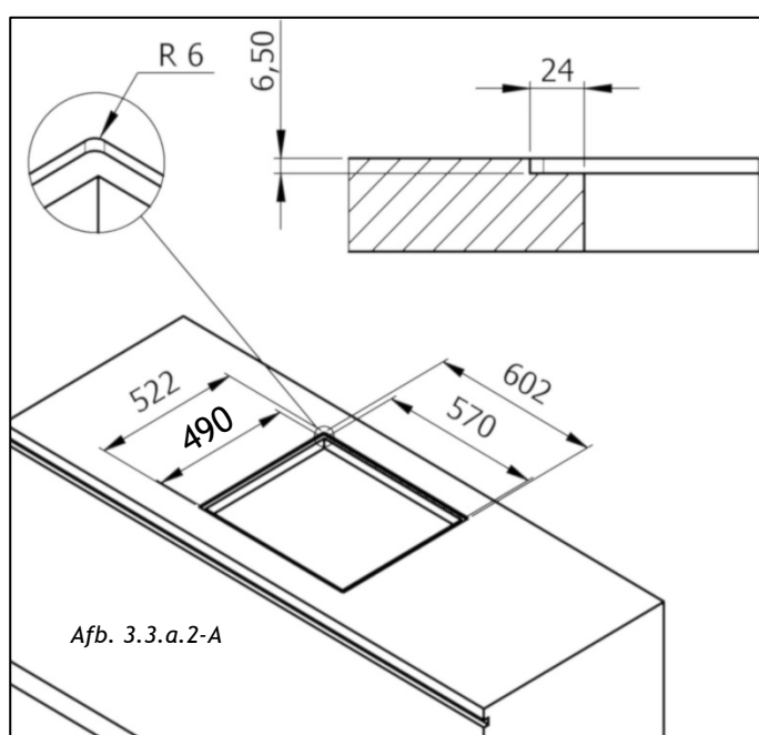
Afb. 3.3.a.2-A -> Kookplaat 60cm.
