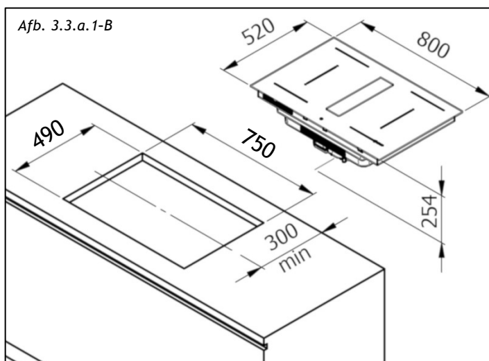
Afb. 3.3.a.1-B -> Kookplaat 80cm.
