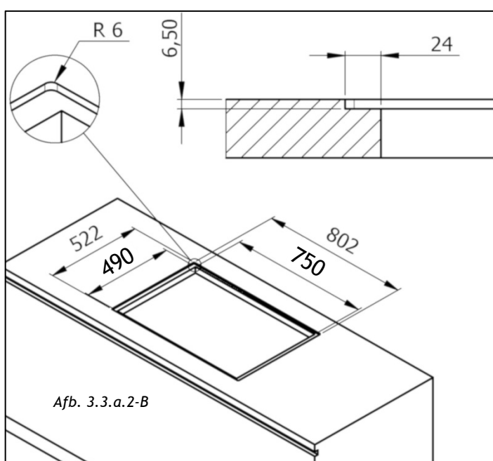
Afb. 3.3.a.2-B -> Kookplaat 80cm.
