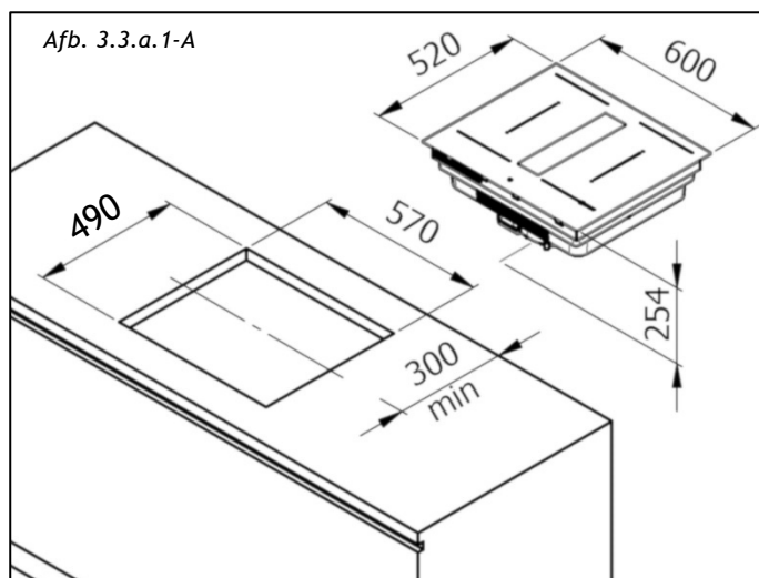
Afb. 3.3.a.1-A -> Kookplaat 60cm.
